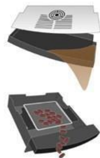
Oppsamlingskuff & Spillbeholder
